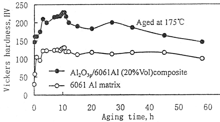
图 3-3 Al_2O_3/6061Al(20\%Vol) 复合材料及基体合金 175°C 时效硬化曲线
